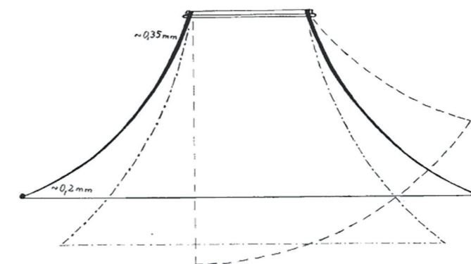
E.シュミットのハンドハンマー加工ベル(リング部分は~0.35mm、ベル端は~0.2mm)
